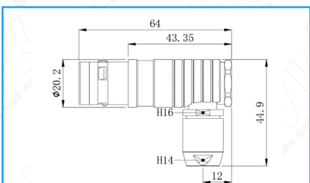
FHG(弯头)
