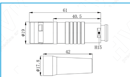
FGG(直头)
