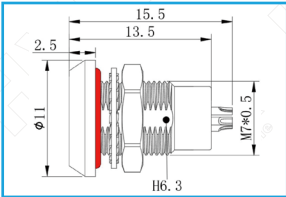
HGG(前面板安装真空密封型插座)
