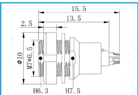
EEG(后面板安装)
