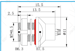
HEG(后面板安装真空密封型插座)
